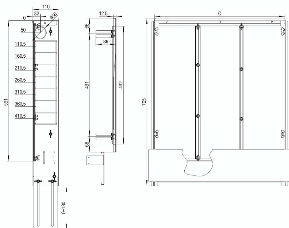
Imag. 9-21 Dimensiuni dulap de distribuție UP C Lățime carcasă interioară
